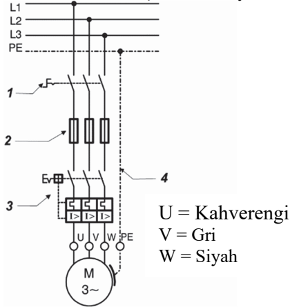
Resim 5-10: Sigorta ve motor koruyucu
