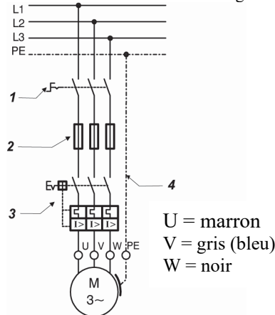
Figure 5-10 : Protection par fusible et protection du moteur
