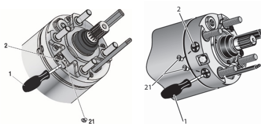
Рисунок 5-2: Двигатель 6", 8", 10"
