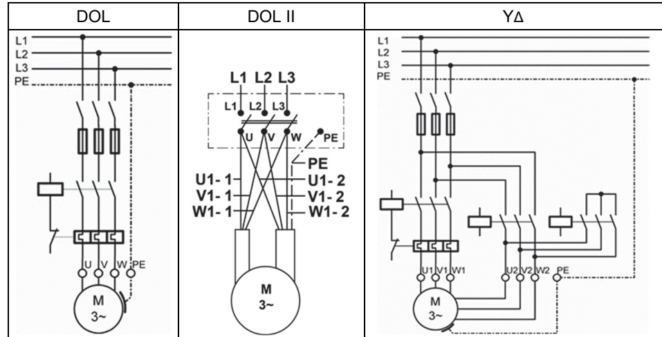
Resim 5-13: Direkt hareket
