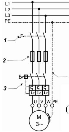
شكل 5 - 10: تركيب المصاهر وحماية المحرك
